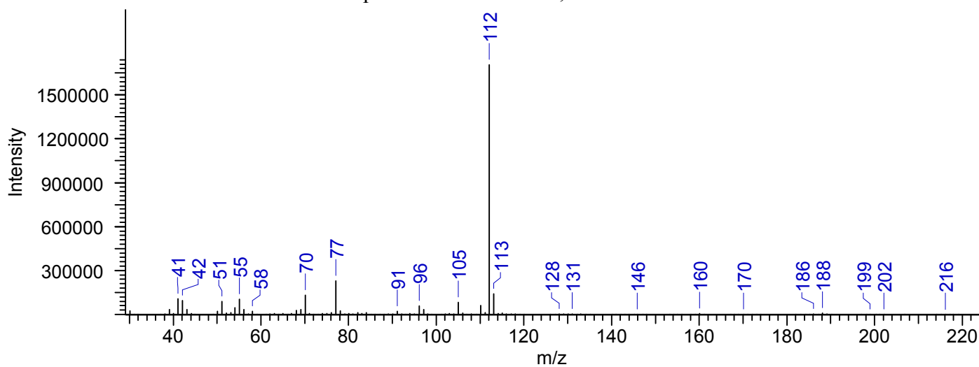
EI Mass Spectrum: \alpha -PBP HCl; Lot ALB-225-2
