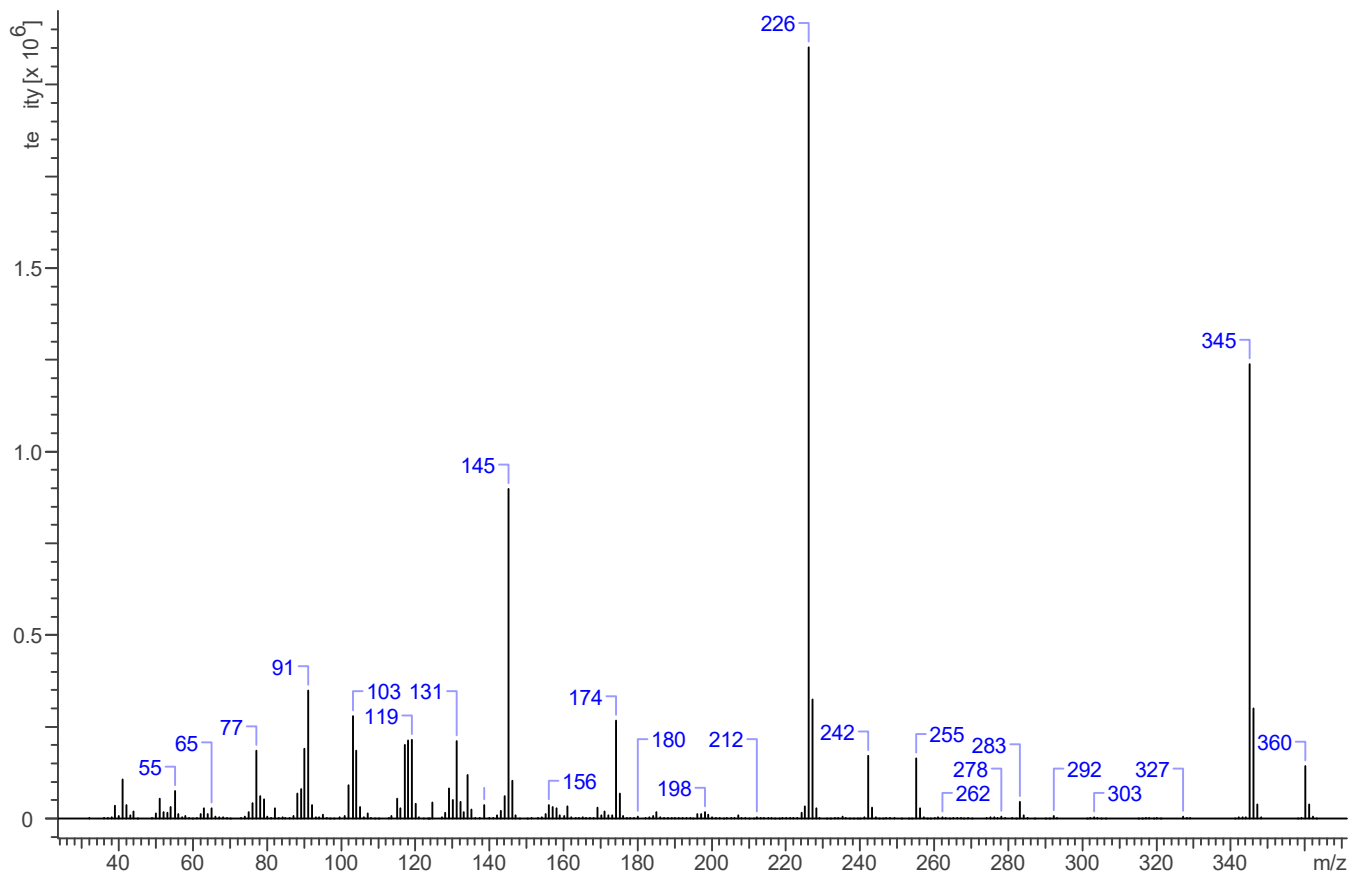
EI Mass Spectrum: 4-cyano CUMYL-BUTINACA; Lot# 0533353-2
